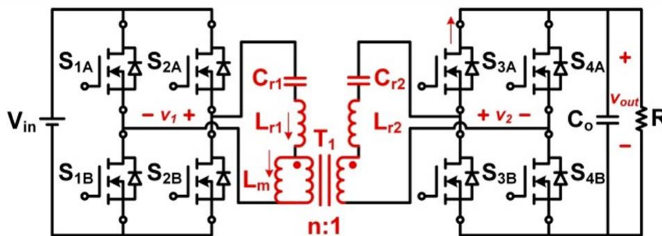
Abbildung 1: Vereinfachtes Ersatzschaltbild der Leistungseinheit eines CLLC-Wandlers [1]
